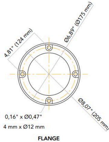
FLANGE
